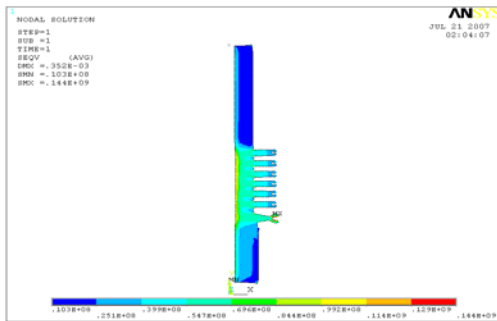
Fig. 12. Von-Mises Stress
