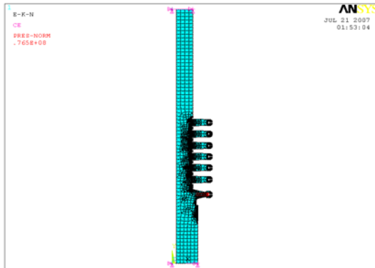
Fig. 11. FE Model
